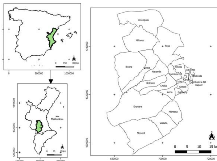
Figura 1. Localidades que integran la agrupación “Municipios del Macizo del Caroig”, pertenecientes a las comarcas de La Ribera Alta, La Costera, La Canal de Navarrés y La Hoya de Buñol, en la provincia de Valencia. Elaboración: B. López-Gurillo-CIDE.
