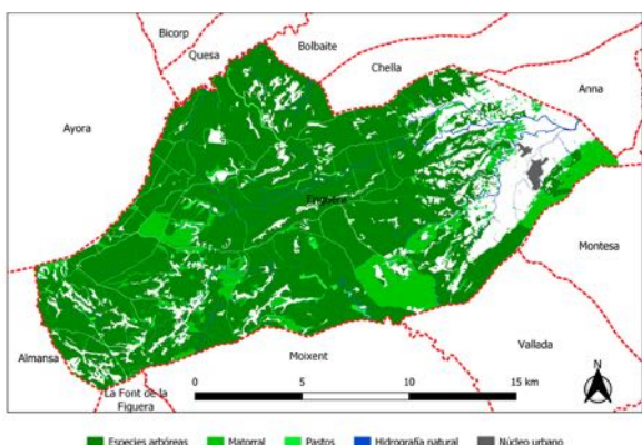
Figura 10. Extensión y continuidad de la masa forestal en el municipio de Enguera, que ocupa un 80% de su extensión total. Fuente: Sede Electrónica del Catastro. https://www.sedecatastro.gob.es/Accessos/SECACCDescargaDatos.aspx . Elaboración: B. López-Gurillo-CIDE.
