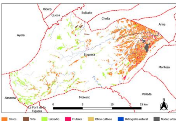
Figura 11. Ubicación actual de los campos de cultivo en Enguera, preferentemente en los valles y suelos más fértiles de la localidad (Clases B y C). Fuente: Sede Electrónica del Catastro. https://www.sedecatastro.gob.es/Accessos/SECACCDescargaDatos.aspx . Elaboración: B. López-Gurillo-CIDE.
