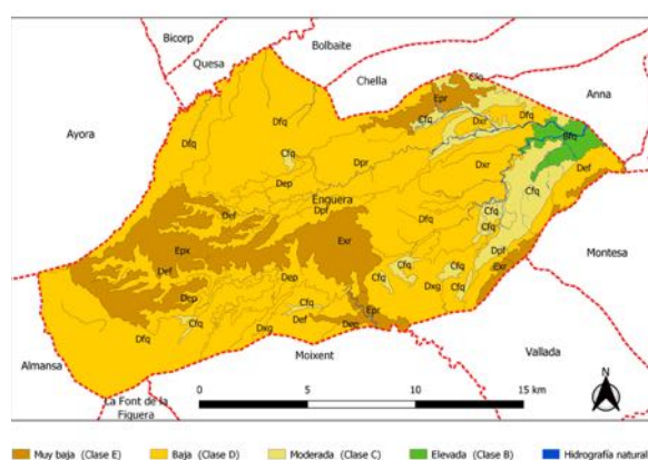
Figura 3. Capacidad de Uso Agrícola de los Suelos, con indicación de las principales limitaciones, en el municipio de Enguera: Características físicas (f); químicas (q); pendiente (p); espesor efectivo de los suelos (x); afloramientos rocosos (r); problemas ligados con la erosión (e); excesiva pedregosidad (g). Fuente: Antolín, C. (Coord.), El suelo como recurso natural en la Comunidad Valenciana. Valencia, 1998. Elaboración para este estudio: B. López-Gurillo-CIDE.
