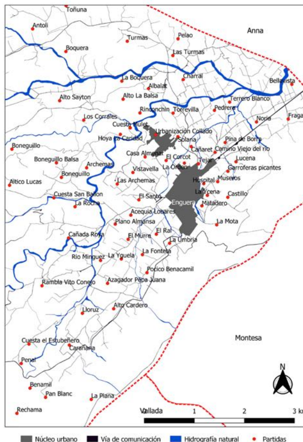
Figura 16. Partidas de cultivo históricas cercanas al núcleo urbano de Enguera. Fuente: Sede Electrónica del Catastro. https://www.sedecatastro.gob.es/Accesos/SECAccDescargaDatos.aspx . Elaboración: B. López-Gurillo-CIDE.
