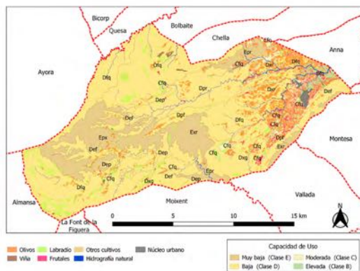
Figura 12. Superposición de la capa de cultivos actuales (Figura 11) a la capa de Capacidad de Uso Agrícola de los Suelos (Figura 3). Elaboración: B. López-Gurillo-CIDE.
