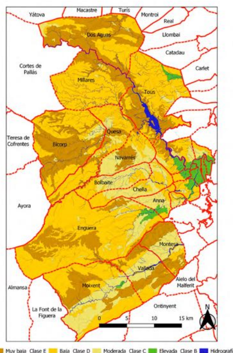
Figura 2. Capacidad de Uso Agrícola de los Suelos de la agrupación “Municipios del Macizo del Caroig”. Fuente: Antolín, C. (Coord.), El suelo como recurso natural en la Comunidad Valenciana . Valencia, 1998. Elaboración para este estudio: B. López-Gurillo-CIDE.
