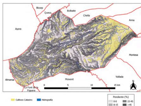
Figura 6.- Ubicación de las partidas rurales actualmente en cultivo: son mayoritarias las situadas en zonas de hasta un 15% de pendiente. Fuente: Centro Nacional de Información Geográfica. Ministerio de Transportes, Movilidad y Agenda Urbana. http://centrodedescargas.cnig.es/CentroDescargas/index.jsp . Elaboración: B. López-Gurillo-CIDE.
