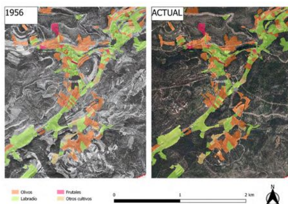
Figura 7. Abandono de campos de cultivo en la zona de Navalón (Enguera), que se evidencia al superponer la capa de cultivos actual a la foto aérea de 1956. Fuente: Centro Nacional de Información Geográfica. Ministerio de Transportes, Movilidad y Agenda Urbana. http://centrodedescargas.cnig.es/CentroDescargas/index.jsp . Elaboración: B. López-Gurillo-CIDE.
